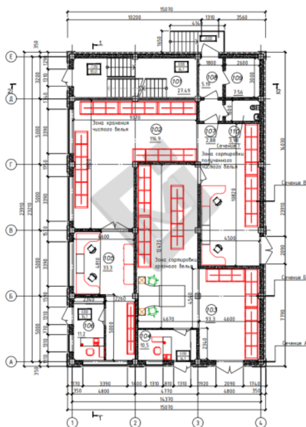
План на отгг 0.000
